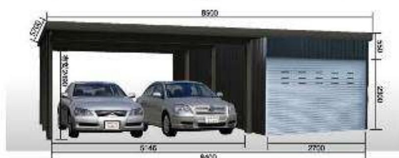
ALTWCPGC (W8920×D5700×H2800)
