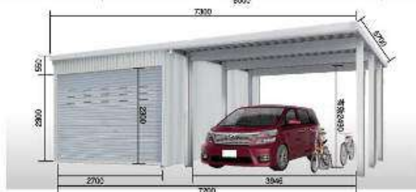
ALWGC (W7300×D5700×H2800)
