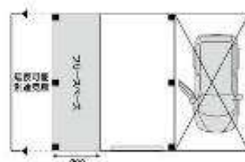
フリースペース+ガレージ+カーポート1台 NL54823SK9HOP-200 (A:5900×D:5400×H:2500)
