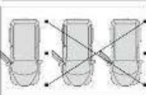
カーポート1台+カーポート2台 HOP-2+1 (A:5900×D:5400×H:2500)
